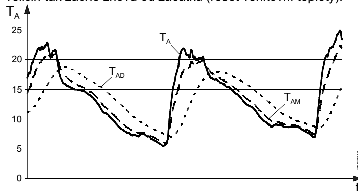
Průběh aktuální, geometrické a tlumené venkovní teploty
